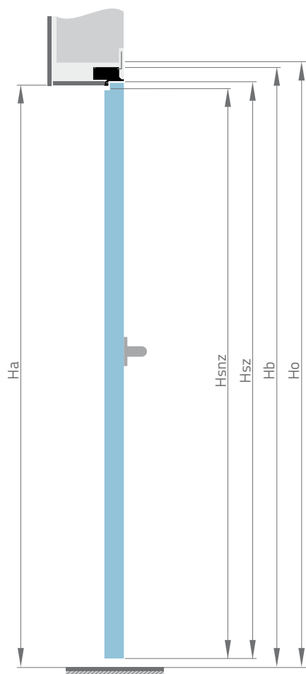
— Drzwi jednoskrzydłowe otwierane standardowo
