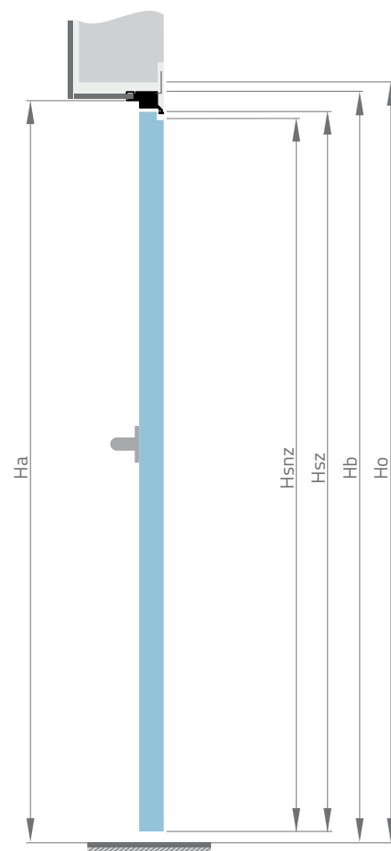
— Drzwi jednoskrzydłowe otwierane przez ościeżnicę
